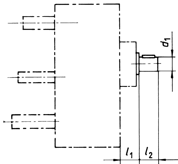
Figure 2 — Arbre d'entraînement
